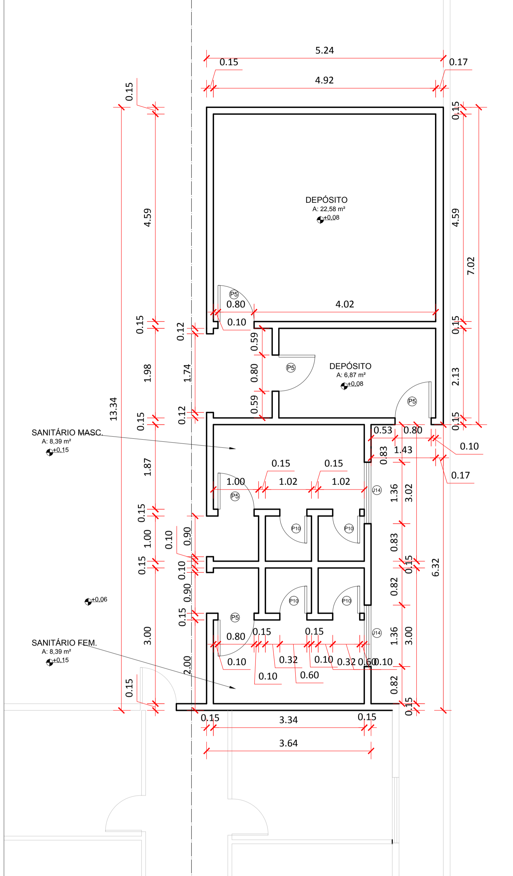
2 PLANTA BAIXA EXISTENTE ESCALA: 1:50
